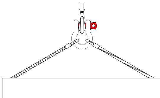
Crochet de levage - Extrémité élingue
