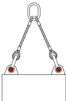
Anneau de levage - Extrémité élingue
