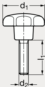
Bouton technopolymère, moulé : 15-27
