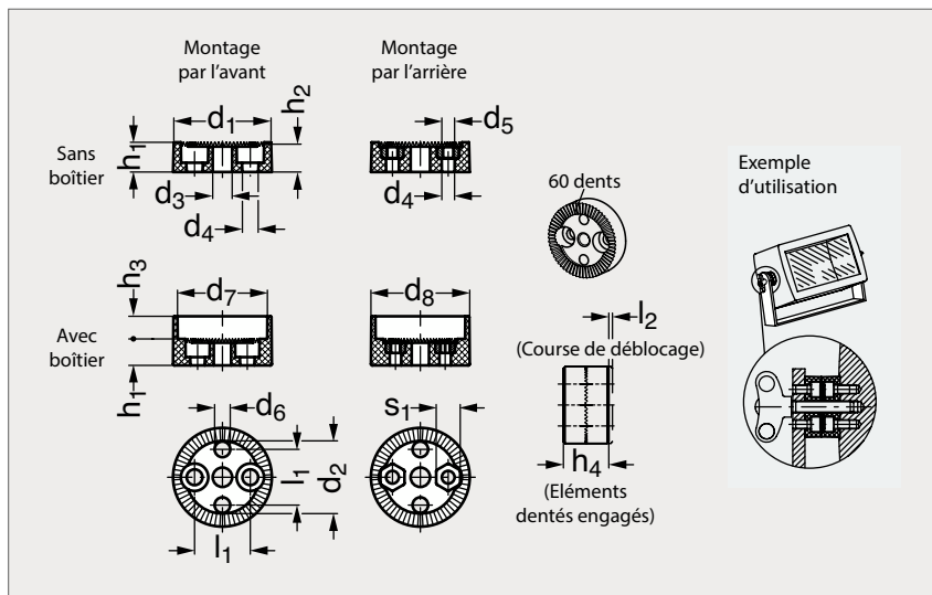
Montage par l'avant, sans boîtier
