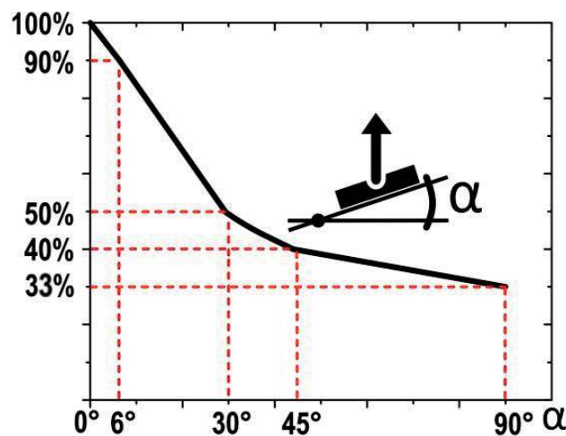
Valeurs de capacité de charge pour l'aimant 18-1452-90
