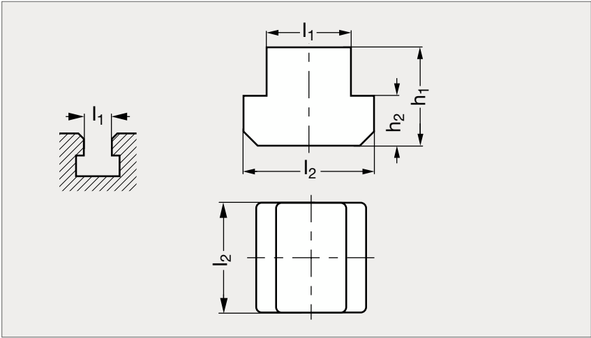
Tasseau DIN 508 23-02 Page 1276
