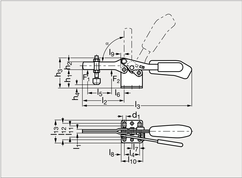
Sauterelle horizontale à bras plein 26-04
