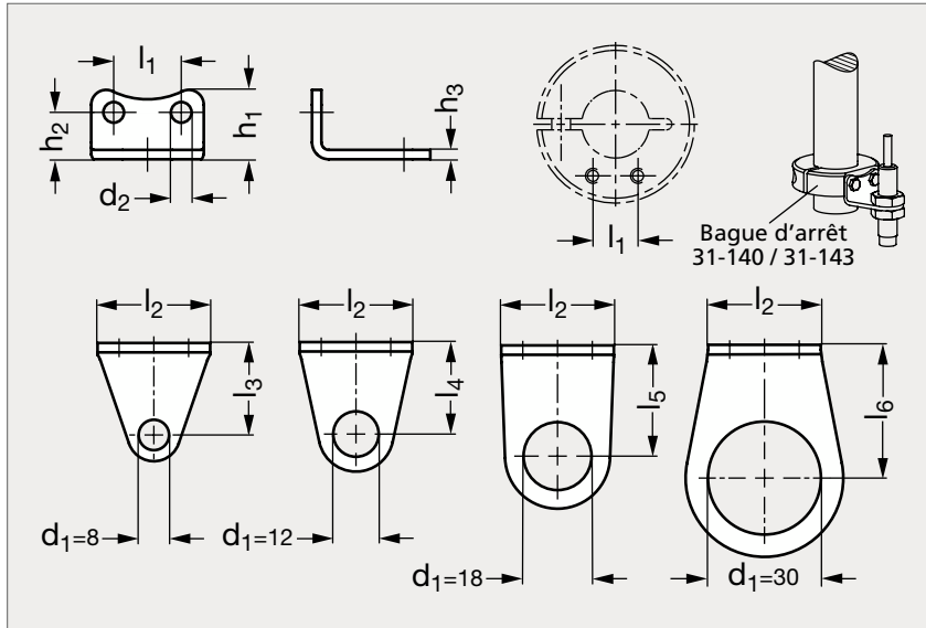
Bague d'arrêt fendue simple 31-140 Page 1506
