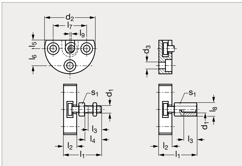
Accouplement à compression radiale 31-80 Page 1545
