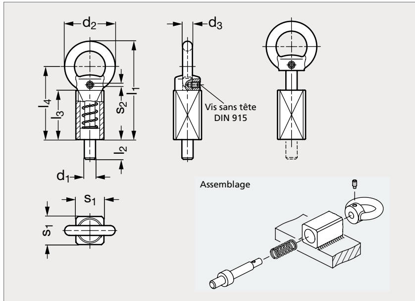
Douille de positionnement 32-39
