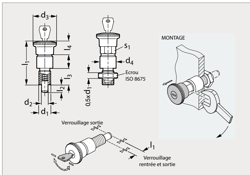
Verrouillage sortie, sans écrou
