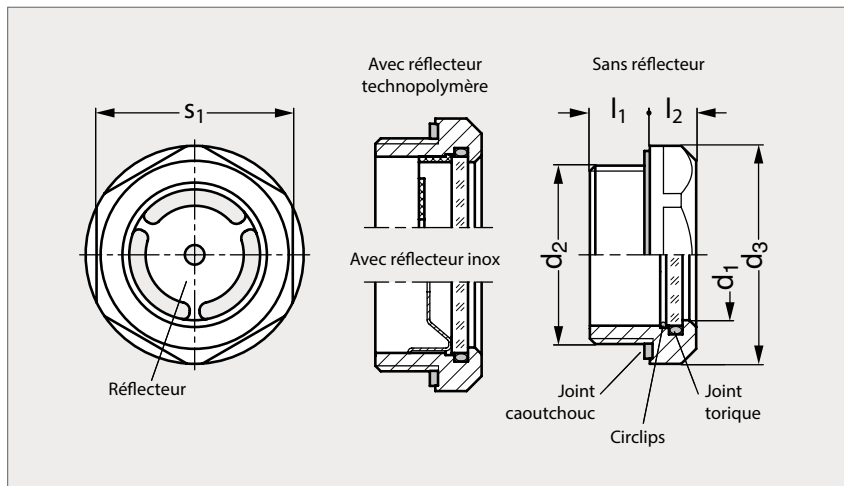
Avec réflecteur technopolymère
