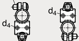
Montage 2 unités linéaires
