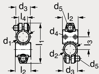
Montage 1 unité linéaire / 1 tube
