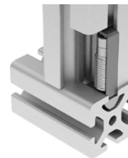
Fixation automatique acier ou inox - Exemple d'application
