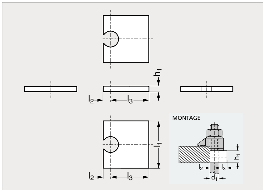
Crapaud fonte, haute résistance, avec logement tête H 95-04
